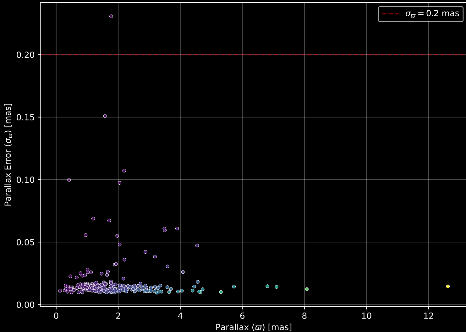
GALAH DR4 Field: [6929] Parallax Quality (n= 292)
