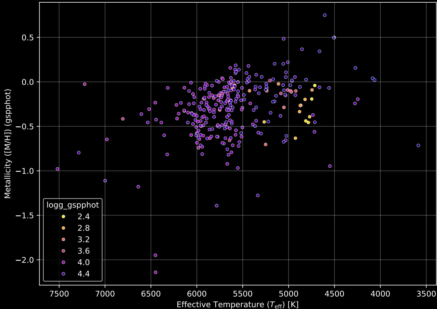
GALAH DR4 Field: [6929] Stellar Population Parameters (n= 292)
