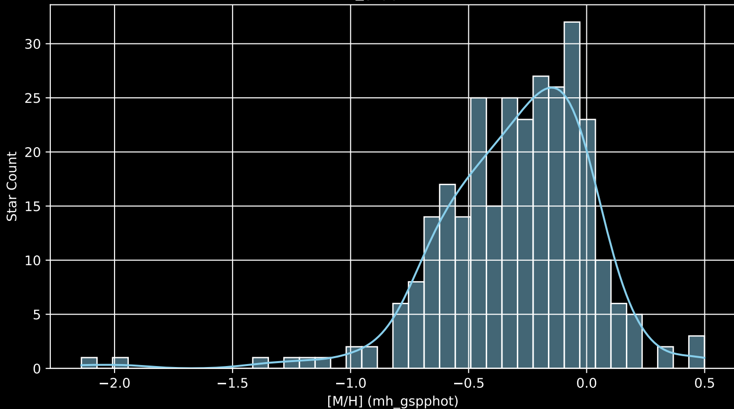
GALAH DR4 Field: [6929] [M/H] (mh_gspphot) (n= 291)
